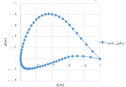
شکل ۷ ایرفویل جدید
