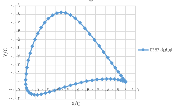
شکل ۳ ایرفویل E387
