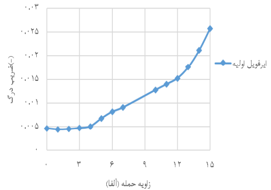
شکل ۶ تغییرات ضریب پسا برحسب زاویه حمله
