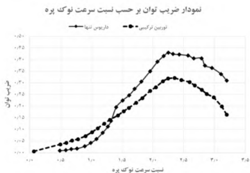
شکل ۴: نمودار ضریب توان بر حسب نسبت سرعت نوک پره برای مقایسه توربین داریوس با هیبریدی [۴۱].
