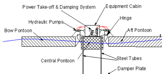
شکل ۴- پمپ موج مک کیب
