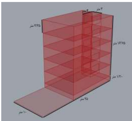
شکل 2 مدل ساختمان‌های شبیه سازی شده با تناسب پایه اولیه برای پاسیوهای نورگیر در پلاگین گرسه‌پایر
