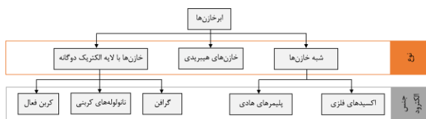
شکل 4 طبقه بندی انواع مختلف ابرخازن‌ها براساس جنس الکترودها
