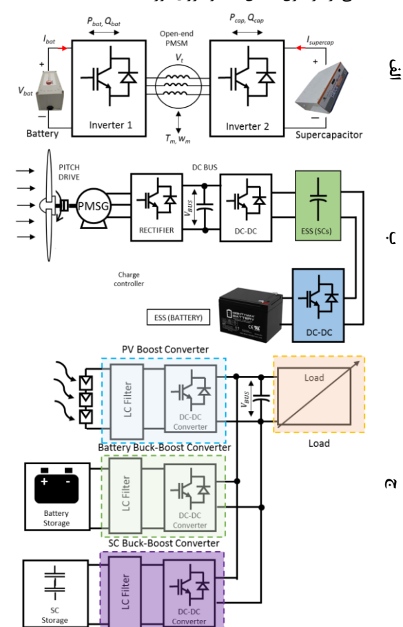
شکل 6 الف - توپولوژی تک مرحله‌ای سیستم ذخیره‌سازی هیبریدی ابرخازن-باتری، ب - سیستم تبدیل انرژی بادی با ذخیره‌ساز هیبریدی ابرخازن-باتری و ج - سیستم تبدیل انرژی خورشیدی با ذخیره‌ساز هیبریدی ابرخازن-باتری [27,28]
