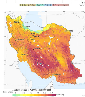
شکل ۱ الف) نقشه‌ی پتانسیل مناطق مختلف ایران در تولید انرژی از پنل‌های فتوولتائیک ب) نقشه‌ی محرومیت مناطق مختلف ایران
