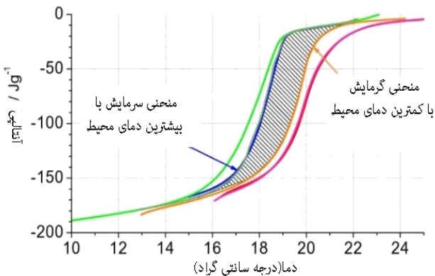
شکل ۱۰ محدوده دما سرمایه‌گذاری و سرمایه‌گذاری در نمودار آنتالپی [۴۰]
