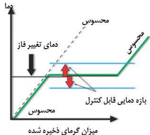
شکل ۱. شماتیک اساس کاری مواد تغییر فازی
