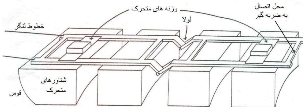
شکل ۷- کلک کوکِرل (یک مبدل هیدرولیکی که در شکل نشان داده نشده است، حرکت نسبی دو کلک را به انرژی قابل استفاده تبدیل می کند).
