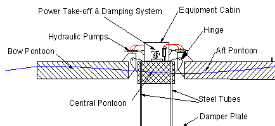
شکل ۴- پمپ موج مک کیب
