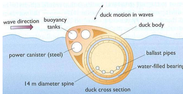
شکل ۶- دوک سالتر (راست) و نحوه تثبیت آن در کف دریا (چپ)
