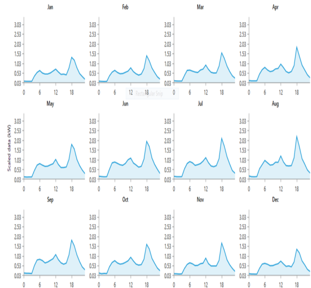
شکل ۴. شبیه سازی بار مصرفی یک خانه با نرم افزار HOMER
