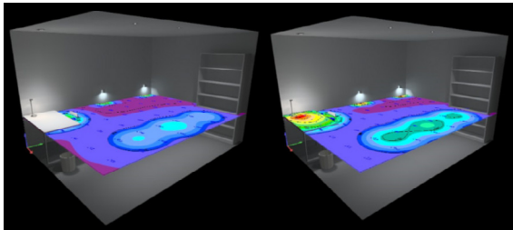
شکل ۷ نمودار فالس کالر ۱ روی سطح کار ۲ اتاق، سمت راست مربوط به فیبر نوری و سمت چپ مربوط به لامپ الکتريکی (خروجی نرم‌افزار دایالوکس)
