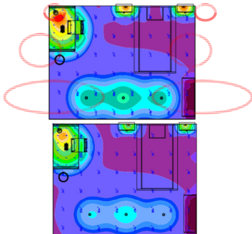
شکل ۹ نمودار فالس کالر پلان اتاق، سمت راست مربوط به فیبر نوری و سمت چپ مربوط به لامپ الکتريکی (خروجی نرم‌افزار دایالوکس)
