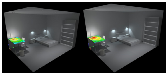
شکل ۸ نمودار فالس کالر روی سطح میز کار، سمت راست مربوط به فیبر نوری و سمت چپ مربوط به لامپ الکتريکی (خروجی نرم‌افزار دایالوکس)
