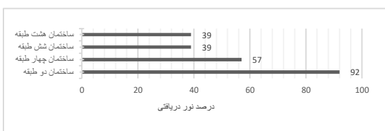
شکل ۱ افت میزان نور دریافتی فضای متصل به چاه نوری با افزایش ارتفاع طبقات بر اساس دی‌لایت اتونومی ۹۲۲ لوکس [۲]
