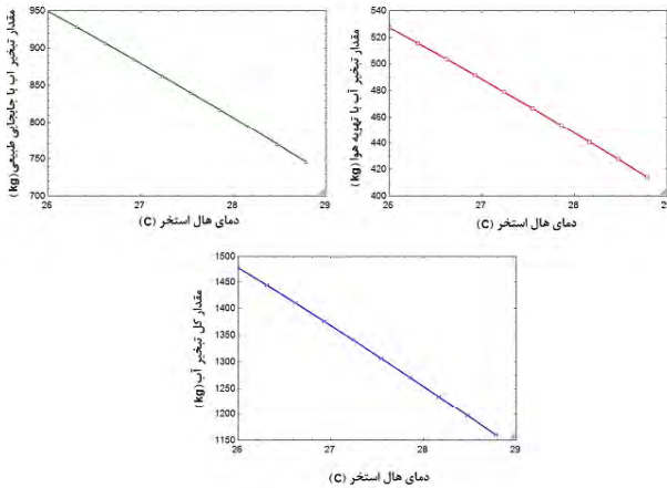
شکل ۵ تاثیر افزایش دمای هال استخر بر مقدار تبخیر آب از استخر
